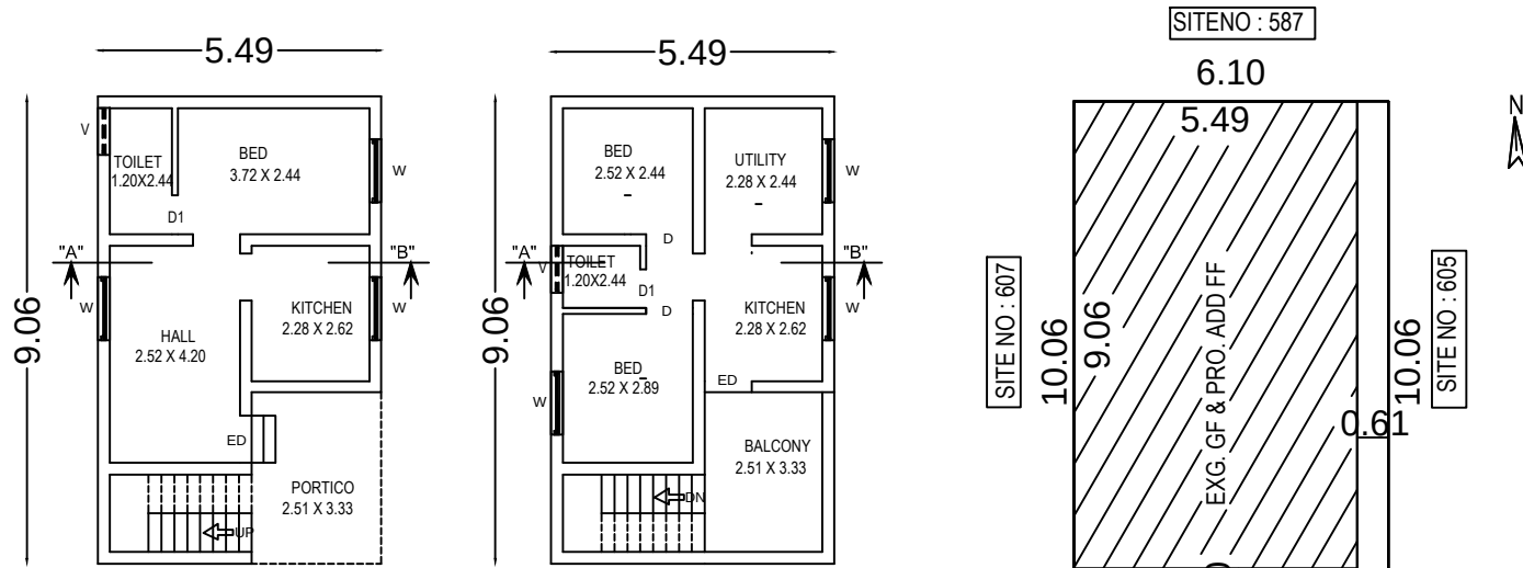
EXG. G.F PLAN
