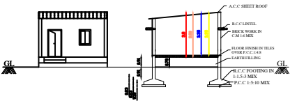
ELEVATION
