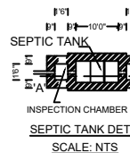
SEPTIC TANK DET SCALE: NTS
