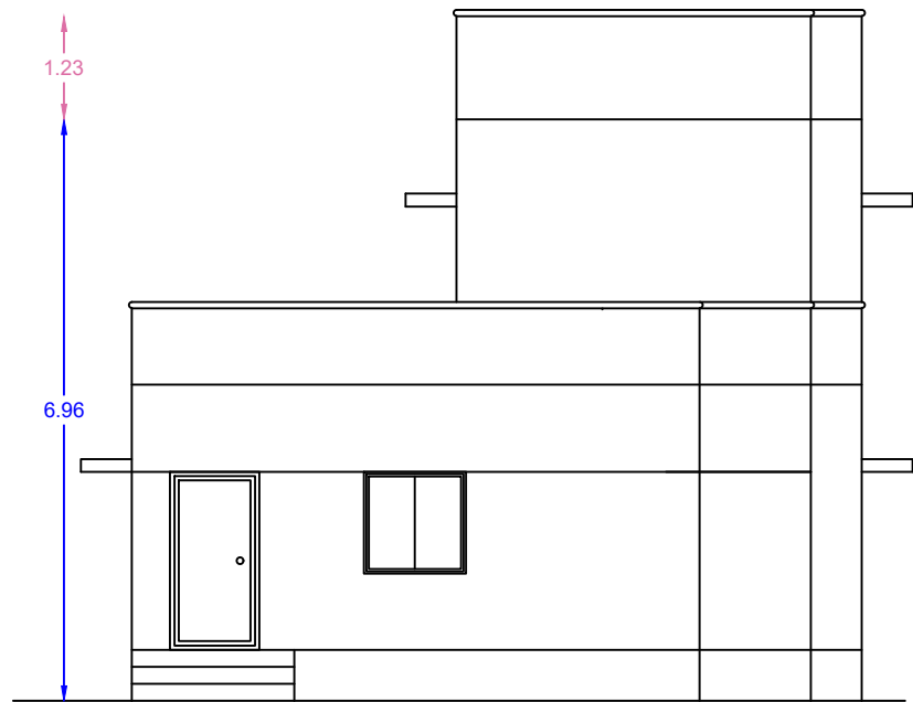
ELEVATION
