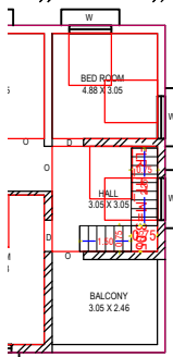
EXISTING BUILDING D.NO. 1/22-C1. D1. FIRST FLOOR PLAN
