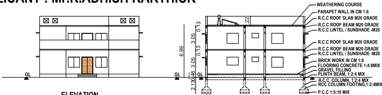
ELEVATION
