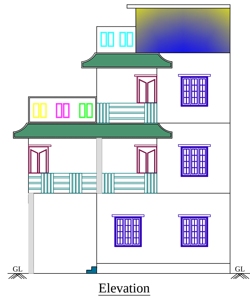
Elevation
