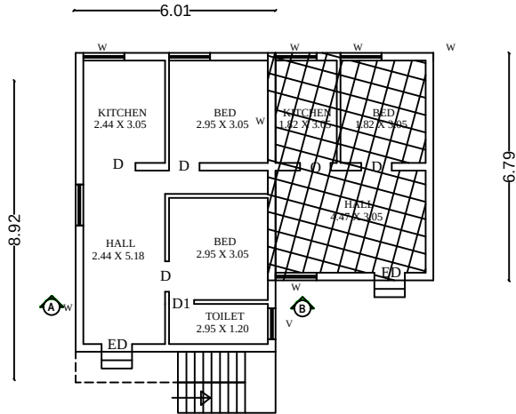
EXG. & PRO. ADD PLAN
