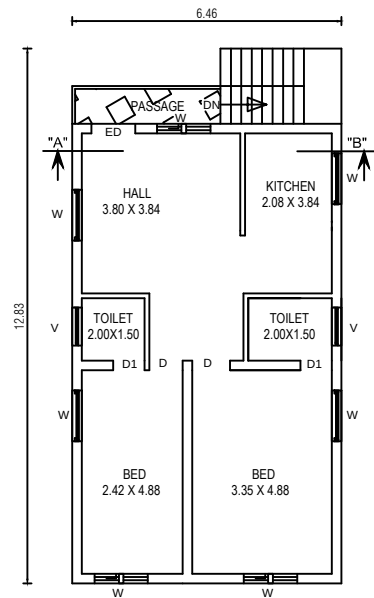
PRO. ADD. F.F PLAN
