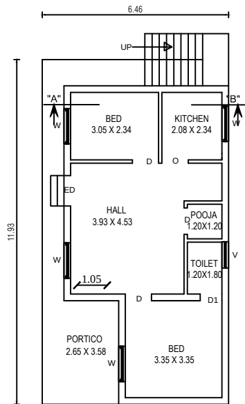
EXG. G.F PLAN
