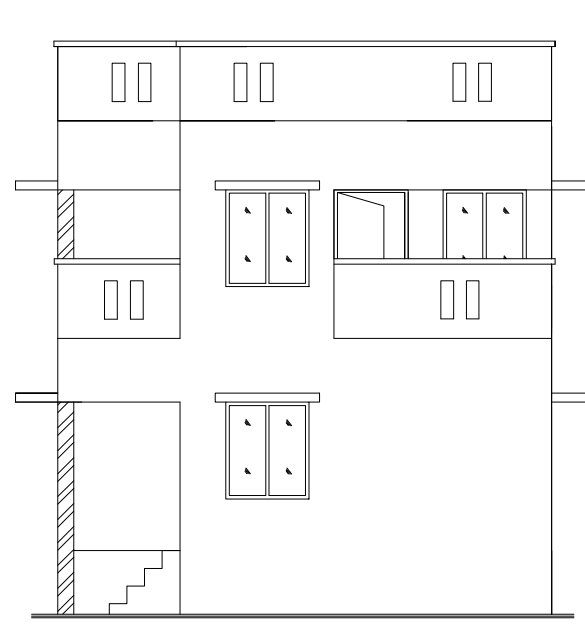
ELEVATION
