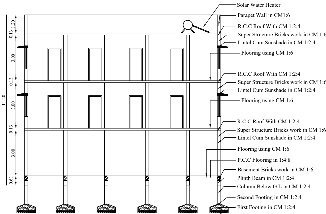
SECTION A-A
