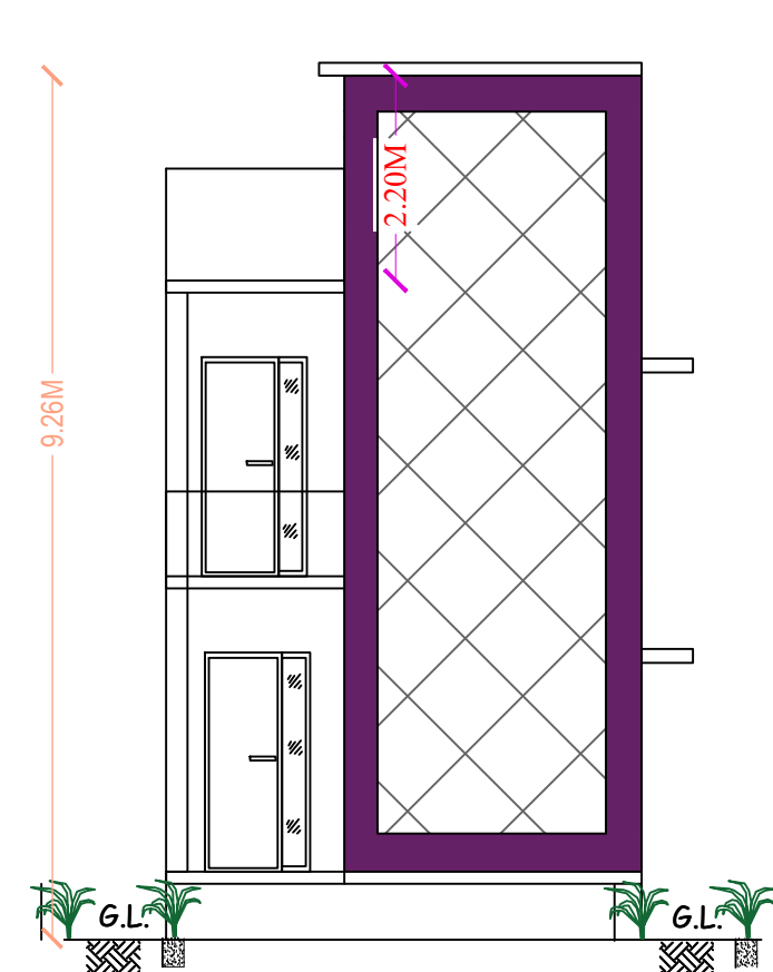
ELEVATION
