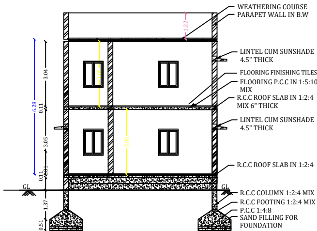
SECTION A-B
