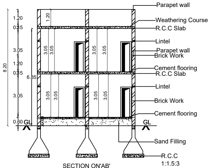
SECTION ON'AB'
