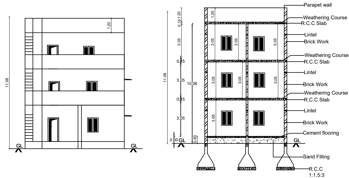
SECTION ON'AB'
