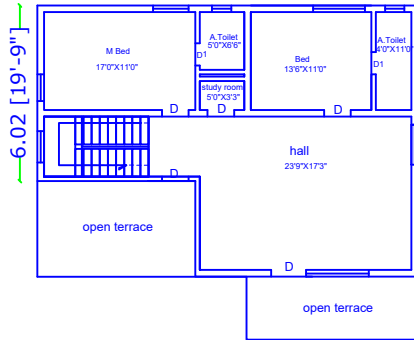
F.F. PRO. BUIL. PLAN
