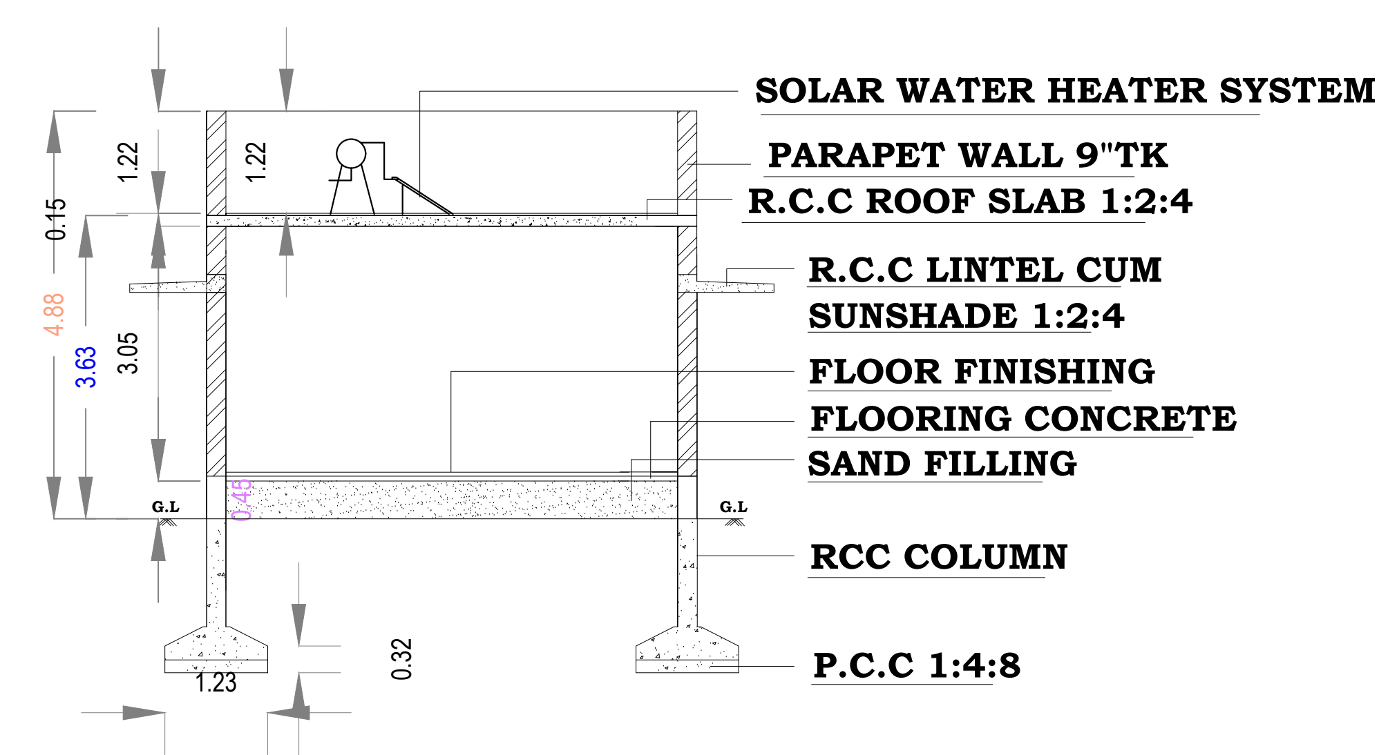
SECTION A-A
