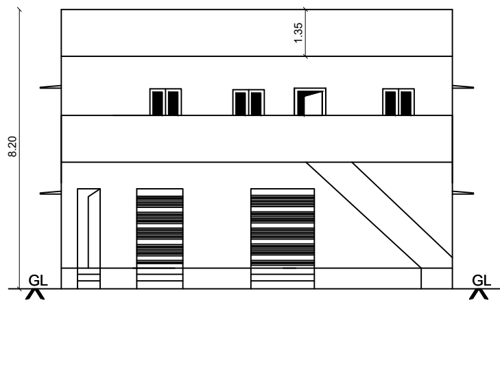
ELEVATION
