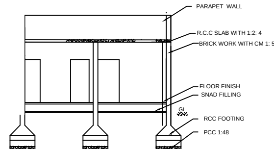
SECTION A-B
