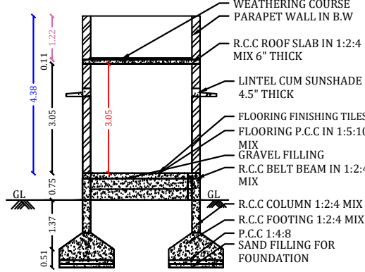
SECTION A-B
