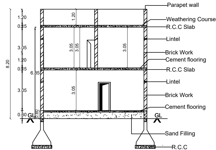
SECTION A-B
