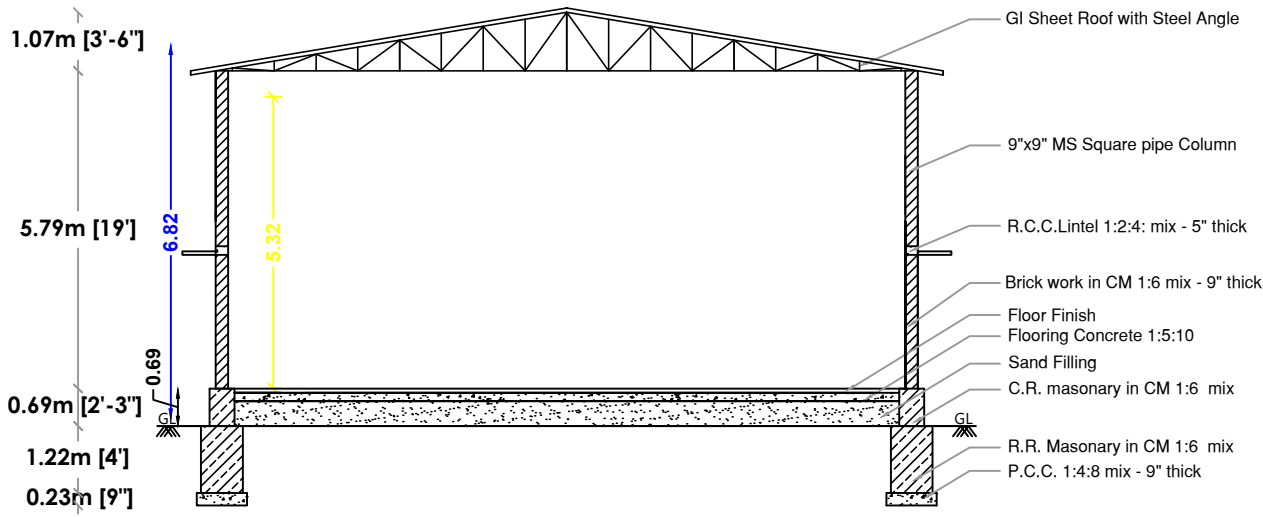
SECTION 'AB'
