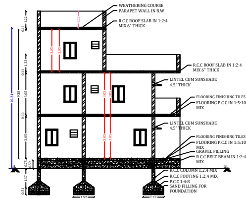
SECTION A-B
