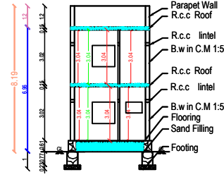
SECTION A-B
