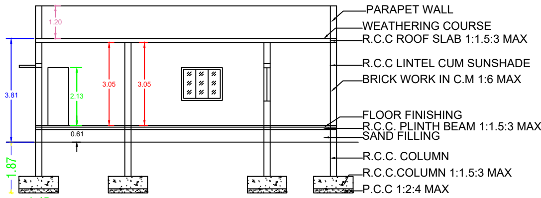
SECTION - AB
