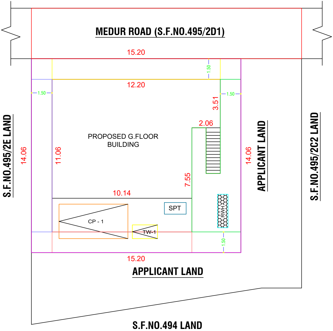
SITE PLAN 1:100
