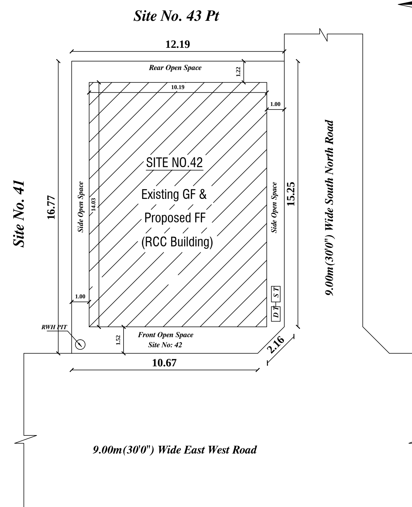
Site Plan (SCALE: 1" = 8' 0")
