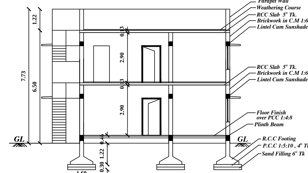
Section On "AB" (SCALE: 1" = 8' 0")
