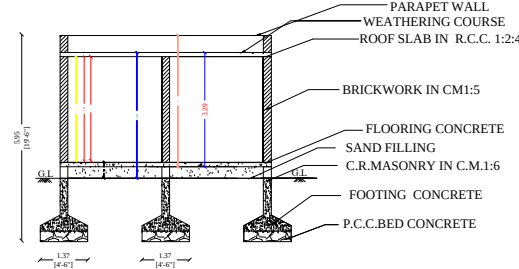
SECTION - AB
