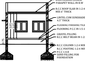
SECTION A-B
