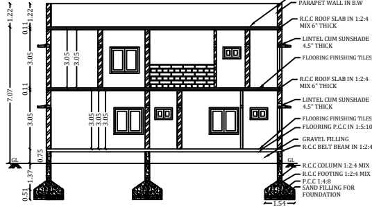
SECTION A-B
