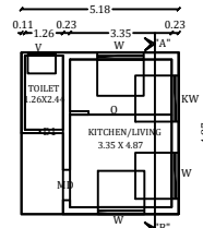
PRO. G.FLOOR PLAN-2
