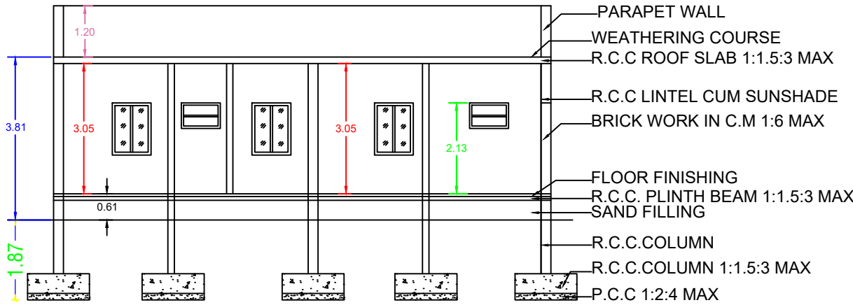
SECTION - AB
