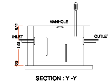
SECTION : Y-Y
