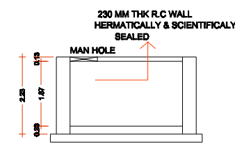
SECTION : X-X
