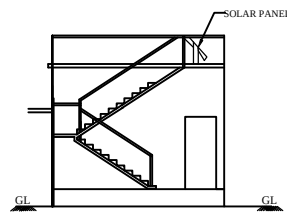
ELEVATION
