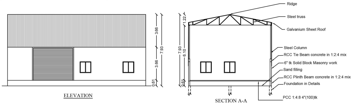
SECTION A-A
