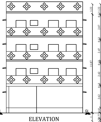
ELEVATION
