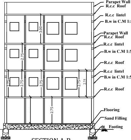
SECTION A-B
