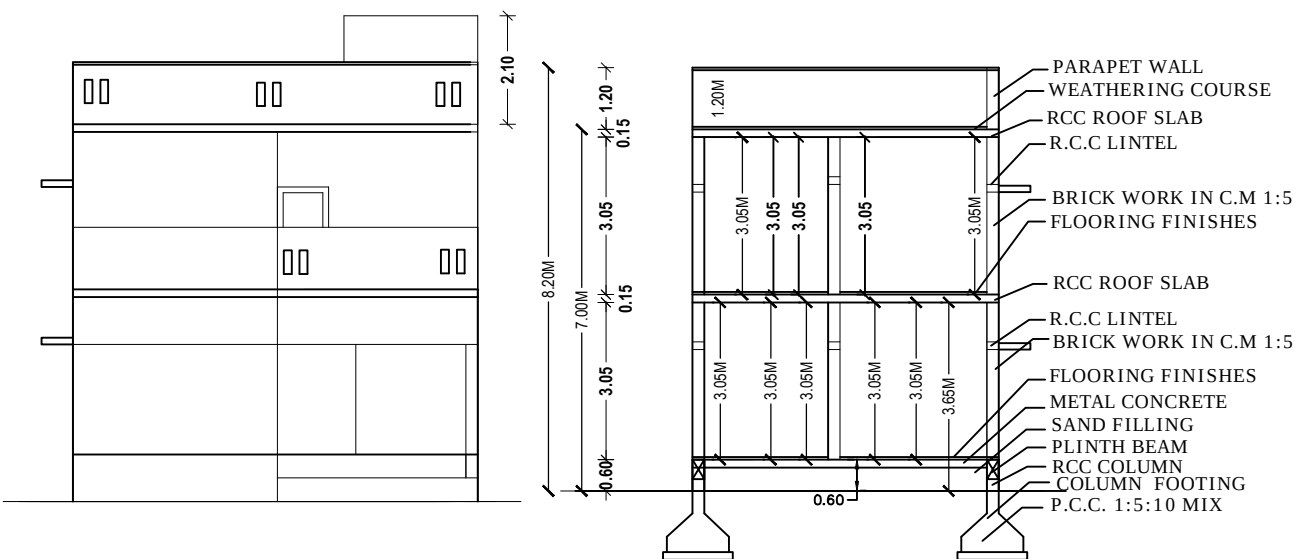
ELEVATION
