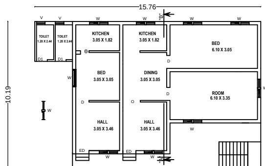
PRO. ALT. & ADD G.F PLAN
