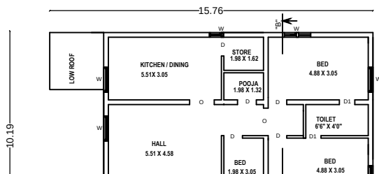
PRO. ALT. & ADD G.F PLAN
