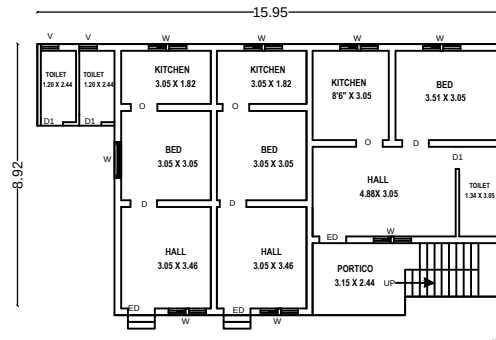
EXG. G.F PLAN
