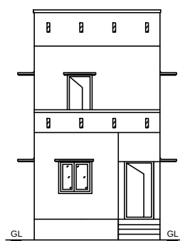
ELEVATION
