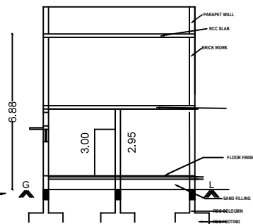
FI ELEVATION
