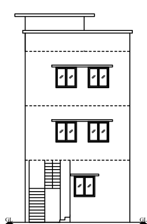
ELEVATION
