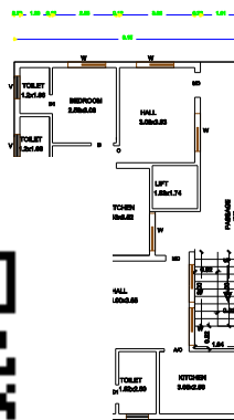
DR PLAN
