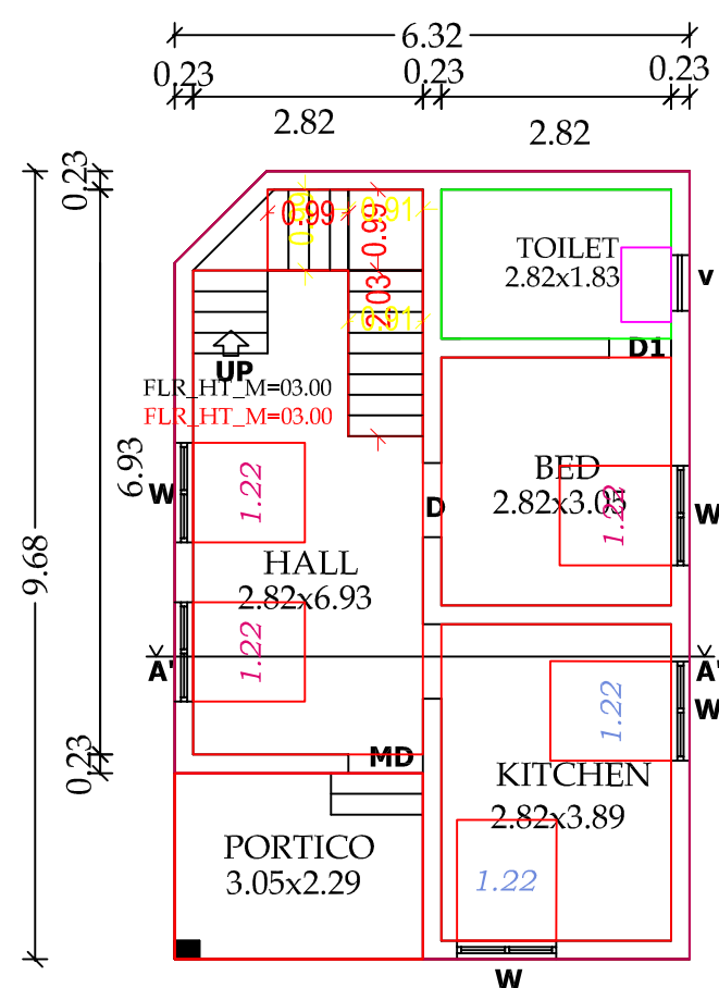
DOOR PLAN
