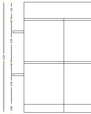
ELEVATION
