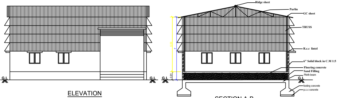
SECTION A-B
