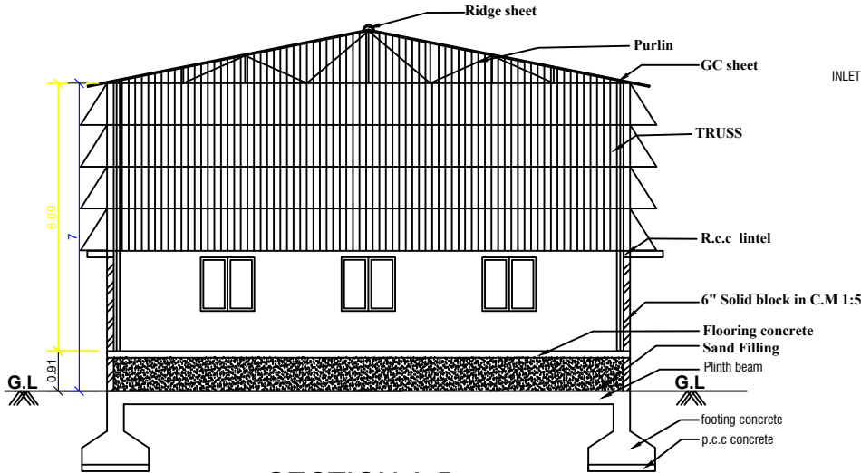
SECTION A-B
