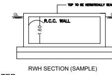
R.W.H SECTION (SAMPLE) R.W.H_CAPACITY_L=2000LTRS
