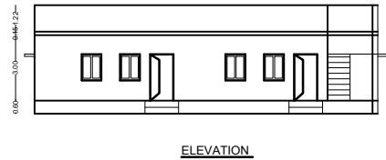
ELEVATION
