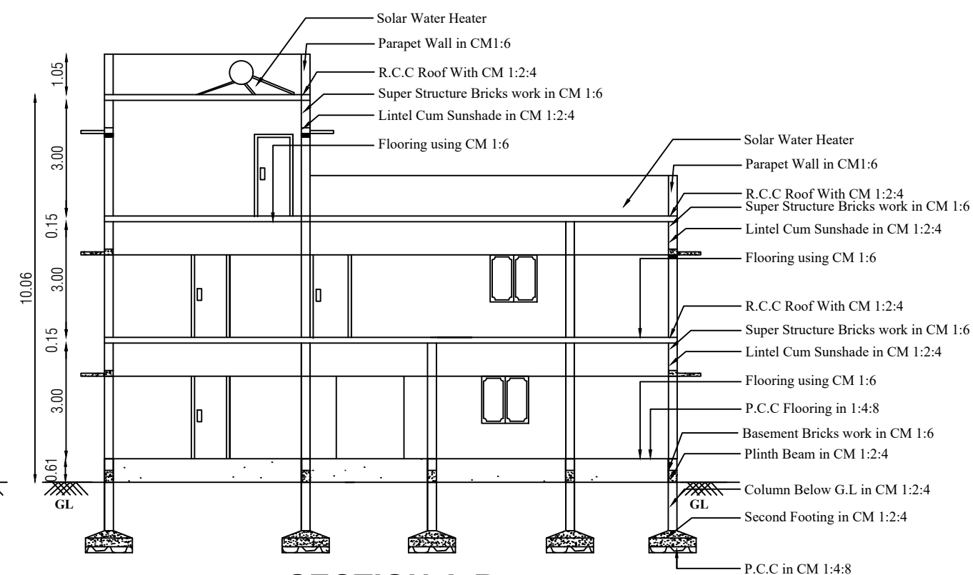
SECTION A-B
