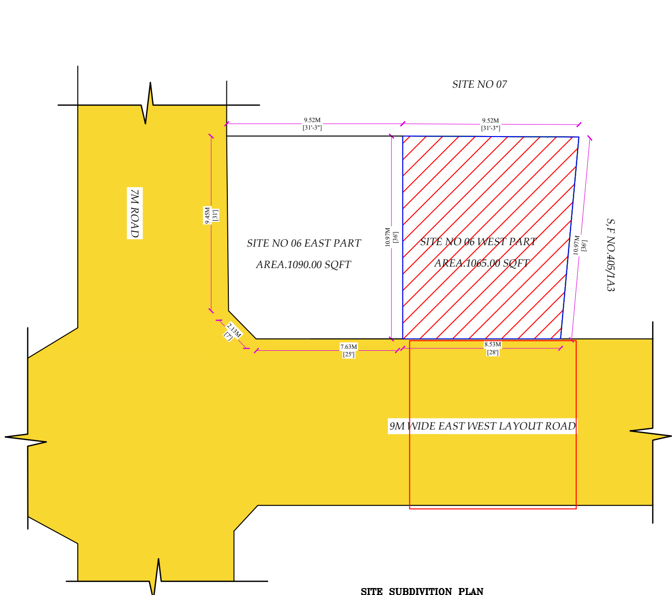
SITE SUBDIVISION PLAN
