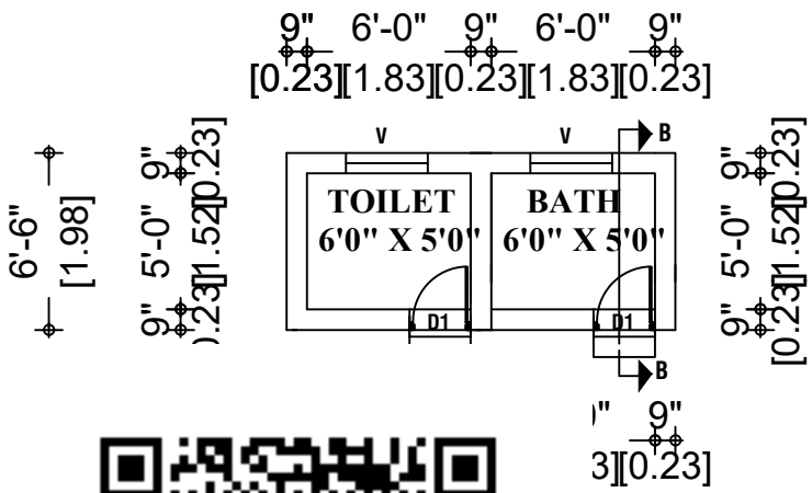
TOILET PLAN
