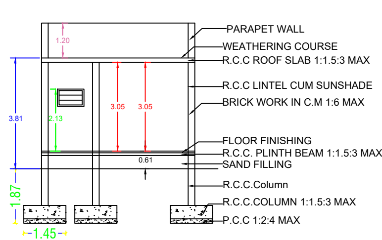
SECTION - AB
