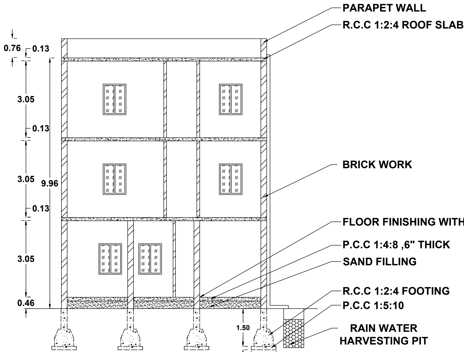
SECTION A-A
